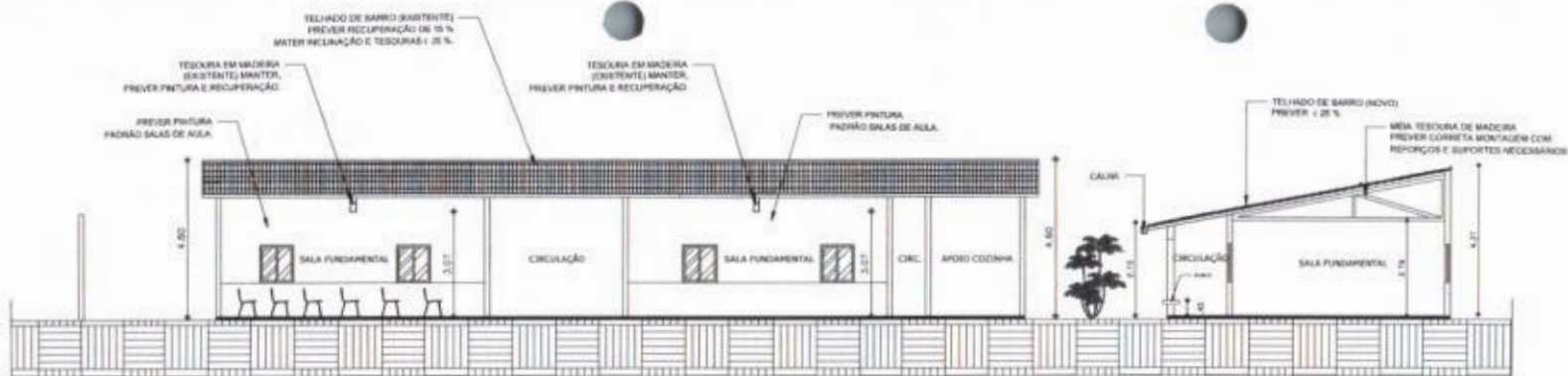
01 CORTE AA 5,00 1,00
