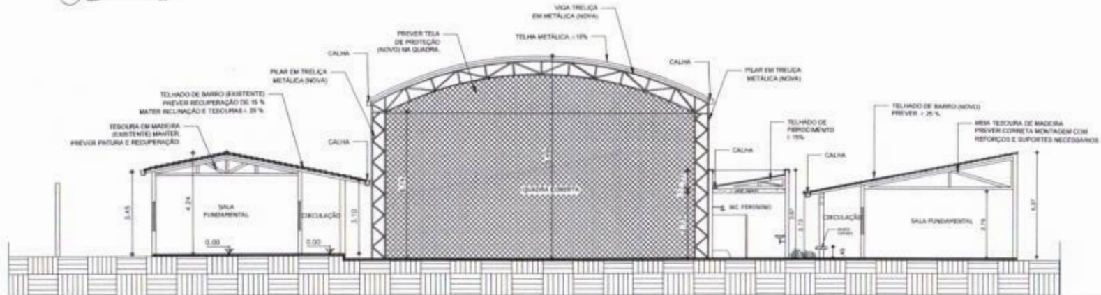
02 CORTE BB 5,00 1,00
