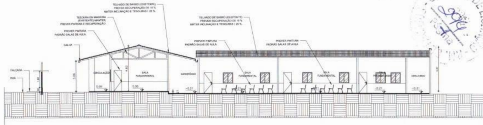
03 CORTE CC 5,00 1,00
