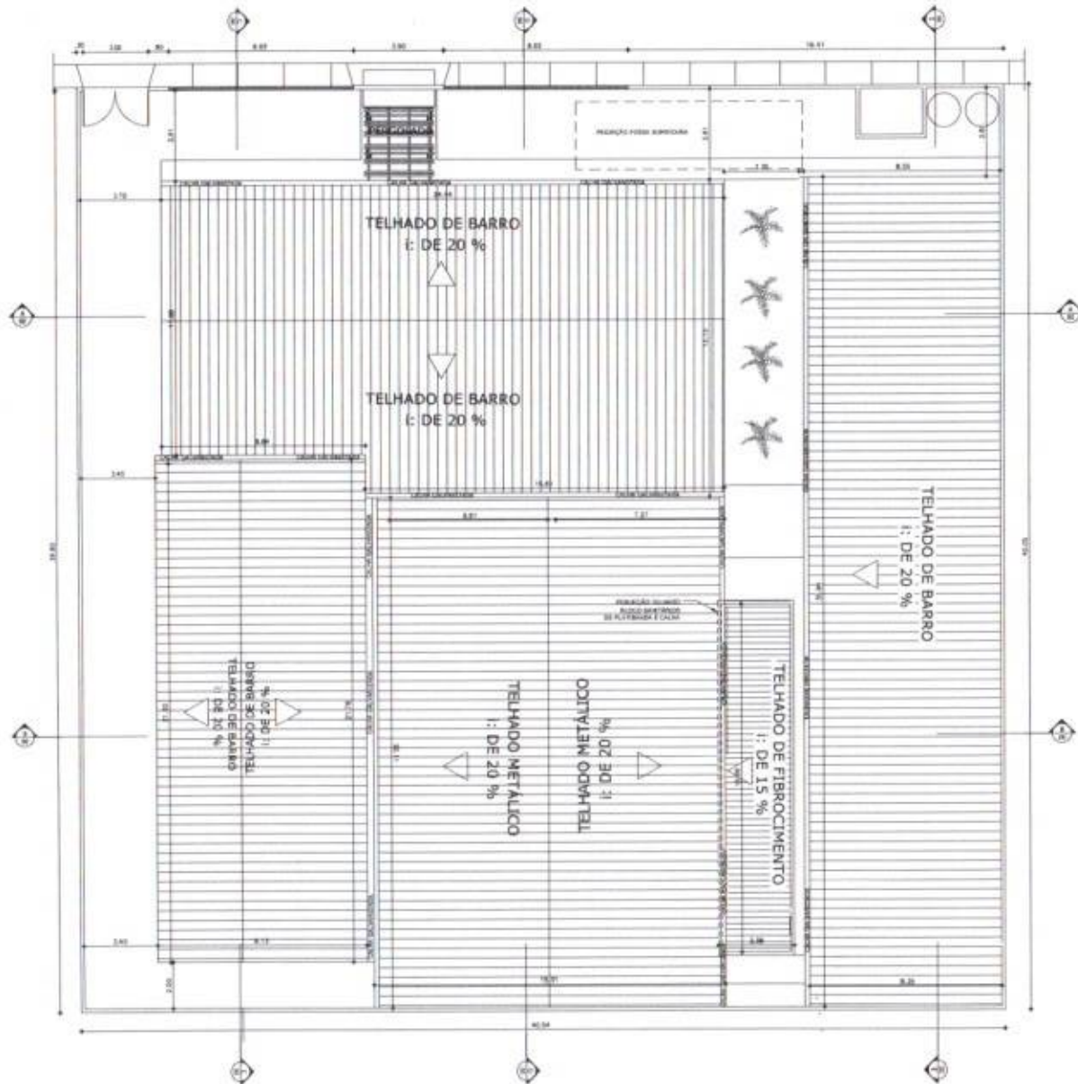
01 IMPLANTAÇÃO + TELHADO
