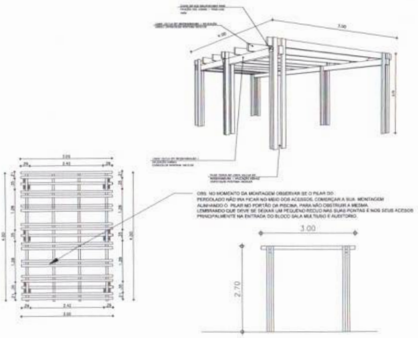
02 DET. PERGOLADO
