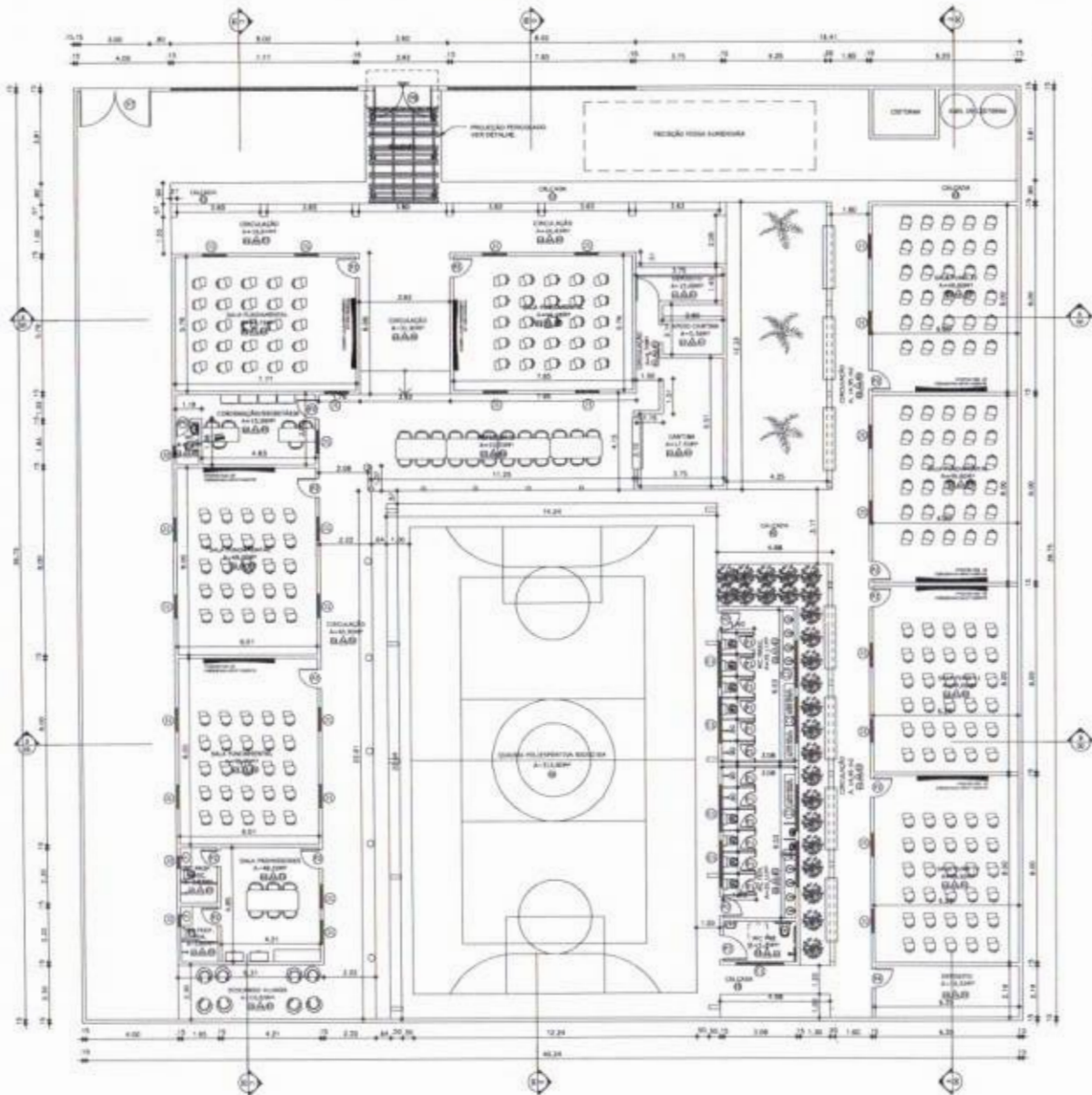
01 PLANTA BAIXA ESCOLA (ITAIPABA) (EXISTENTE)
