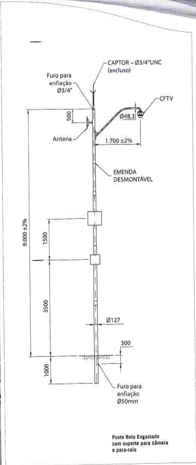
Poste Especial Produzido conforme projeto P.M.S.P. Avenida Paulista - São Paulo
