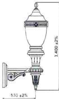
Luz de Parede SP 756
