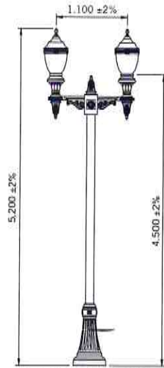
PDR 843B Q-20 / 45L G
