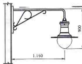
Encaixe de 20,10 mm + ND 220
