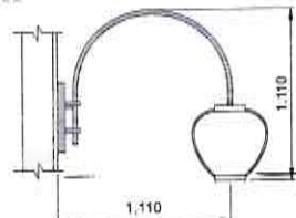
Encaixe de 31,75 mm + ND 236
