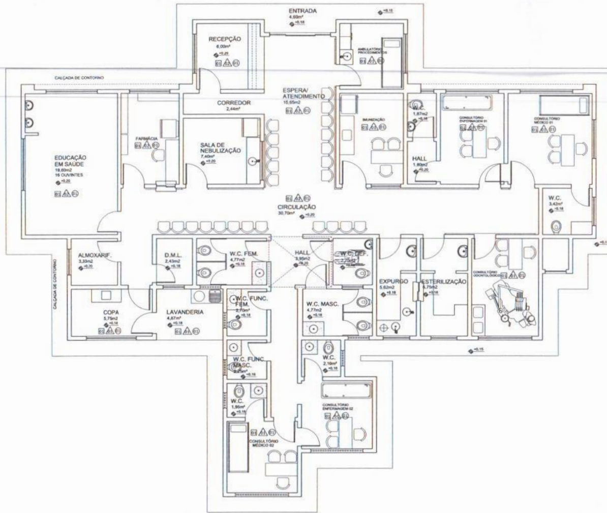
01 PLANTA BAIXA LAYOUT ESCALA 1/750
