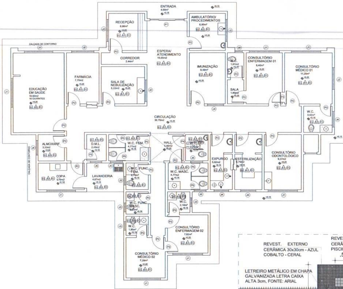
01 PLANTA BAIXA PROPOSTA ESCALA 1/50
